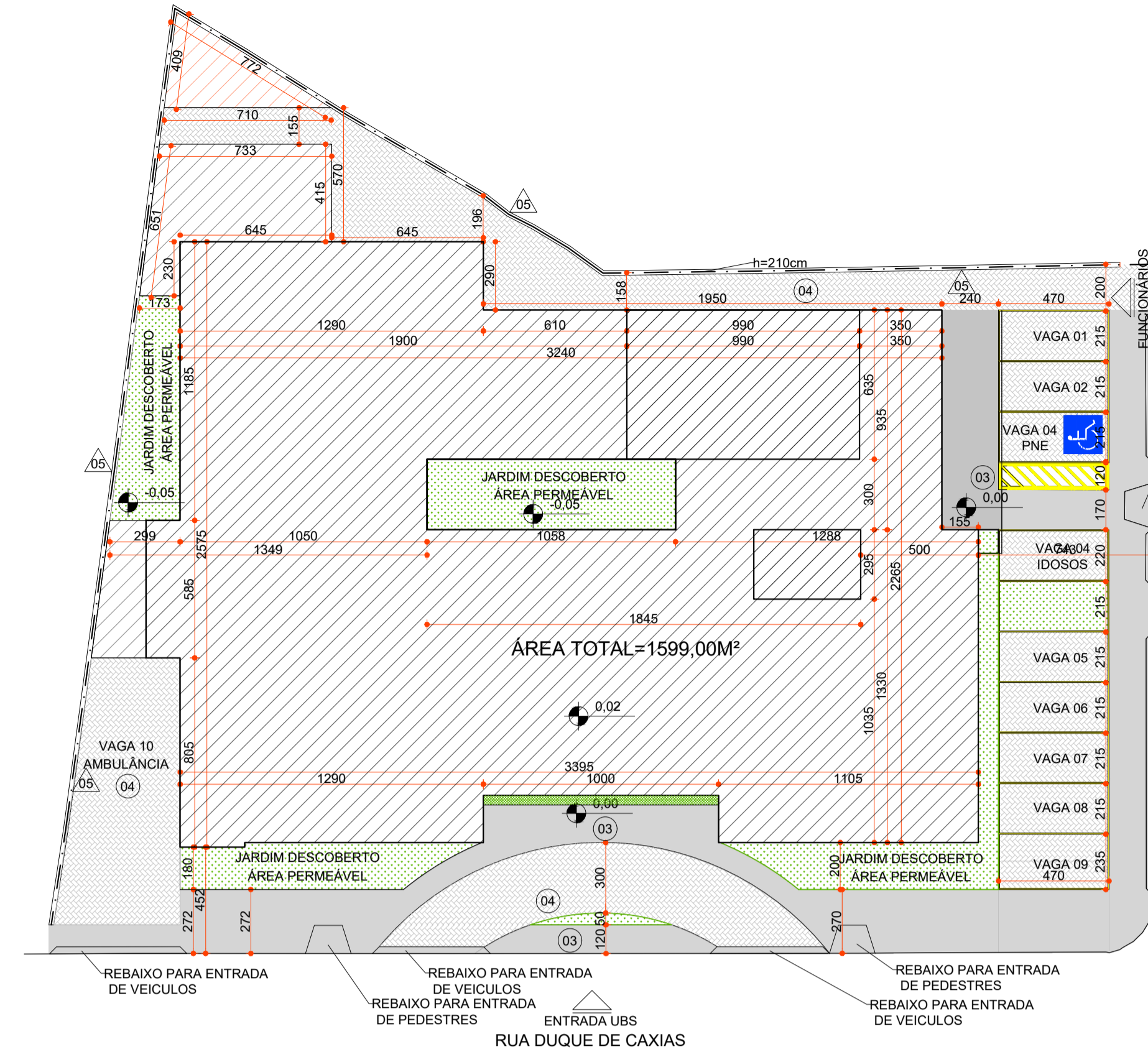
IMPLANTAÇÃO ESCALA 1:200
