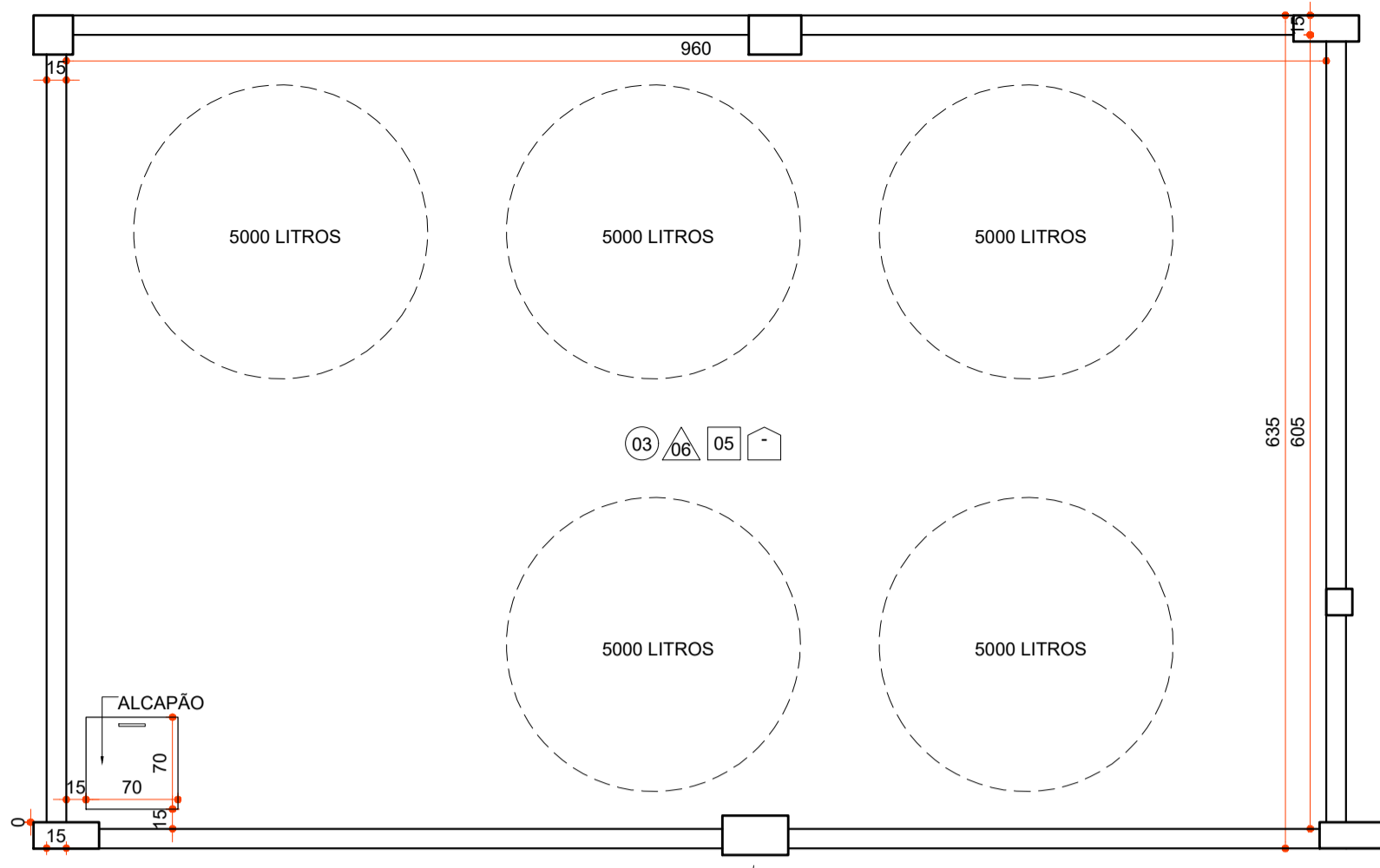
PLANTA DE CAIXA D'ÁGUA ESCALA 1:50
