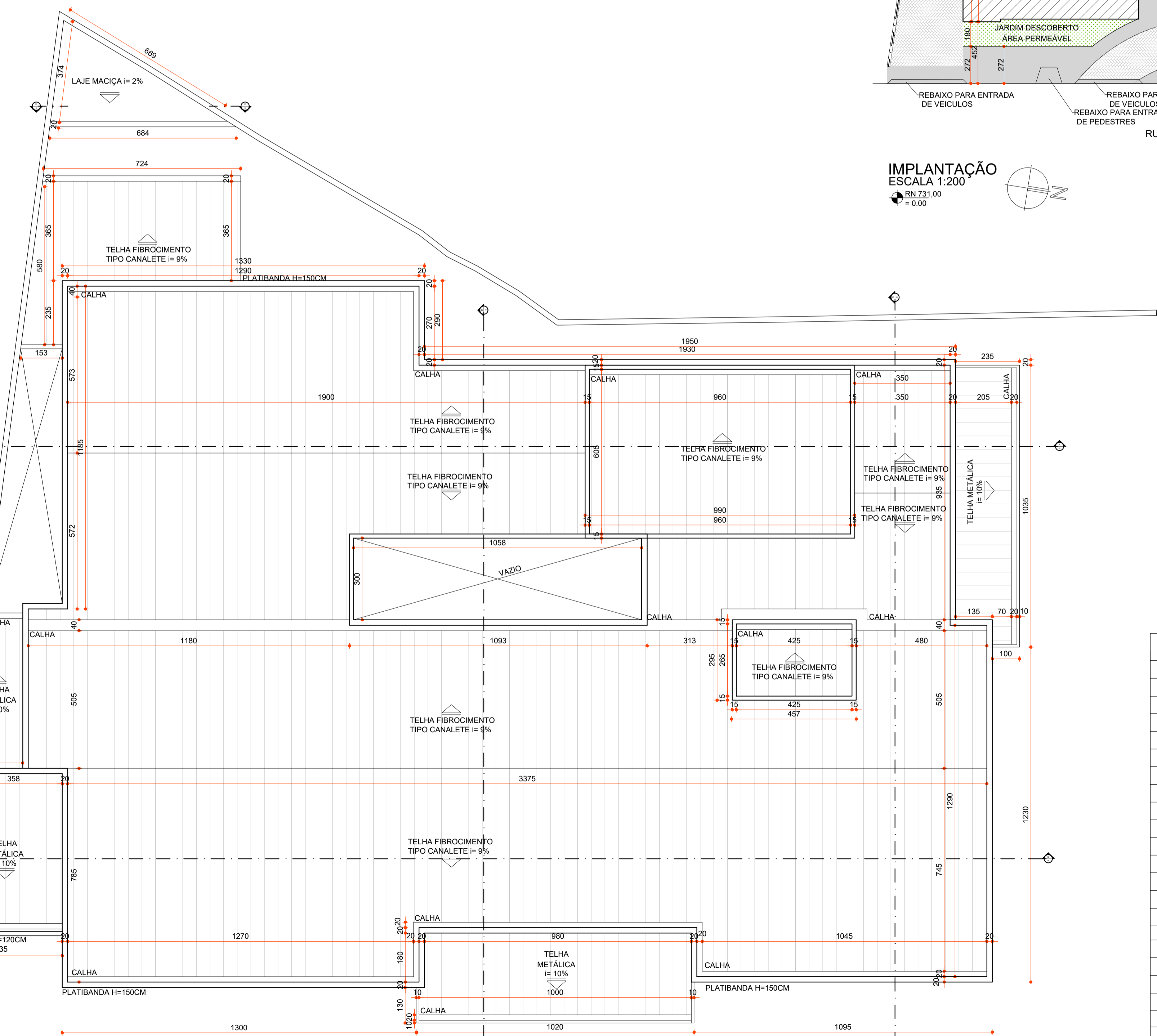
COBERTURA ESCALA 1:100
