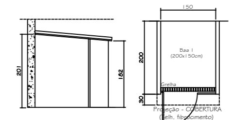
Modelo de baia - Corte e planta
