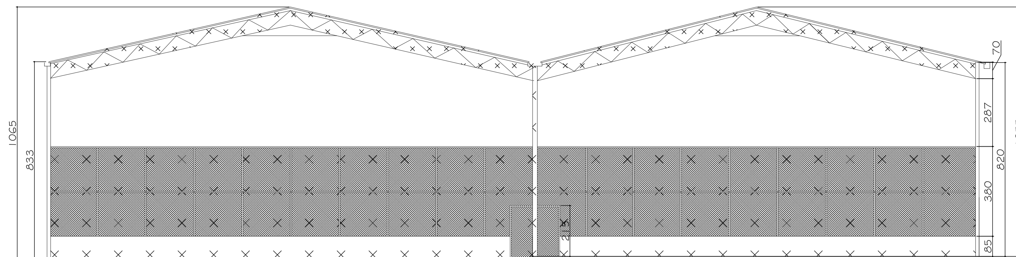
4 ELEVÇÃO DE DEMOLIÇÃO – QUADRA E VESTIÁRIO Esc. 1:100
