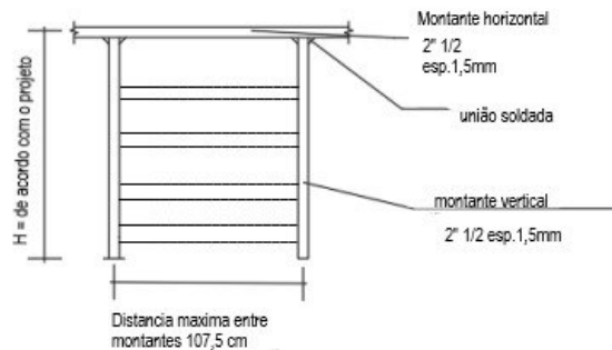
Figura 1: Esquema e estrutura do guarda corpo
